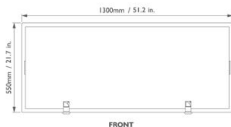
ламинарный поток
